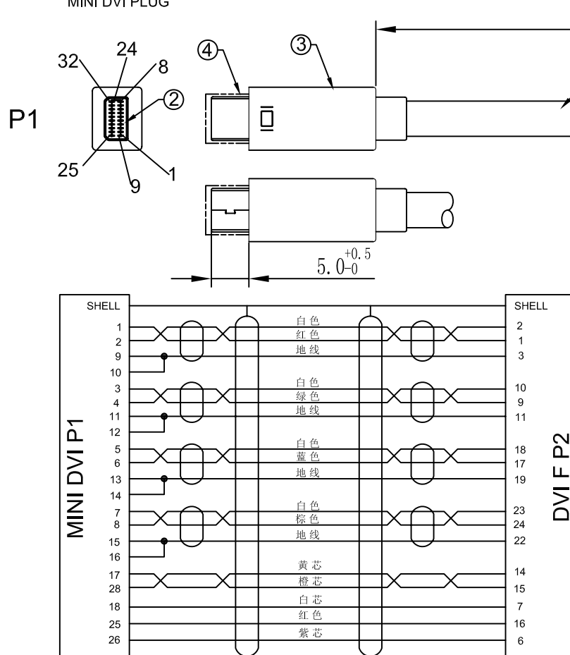
MINI DVI PLUG
